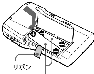
単4形乾電池2本
