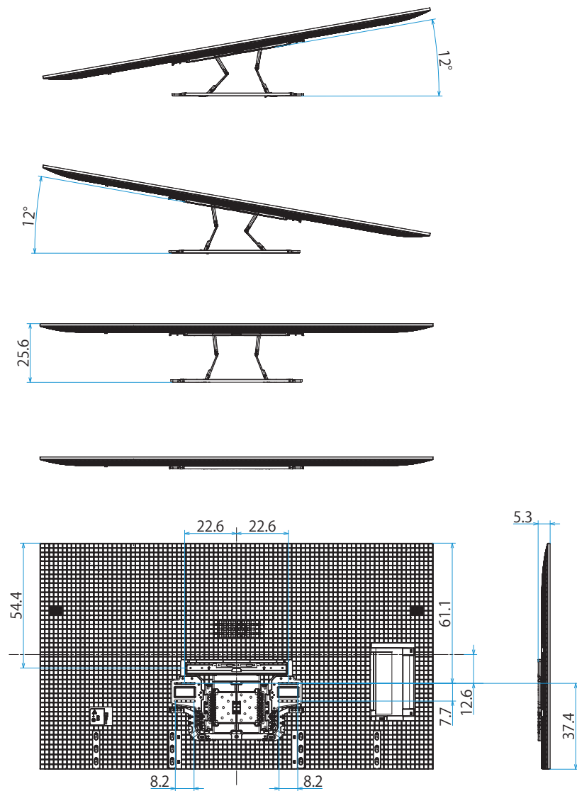
壁掛けブラケット装着時 (SU-WL900/スリム)
